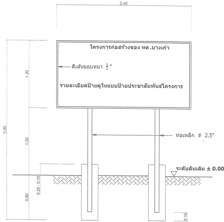
แบบแสดงด้านหน้าป้าย มาตราส่วน 1 : 25
