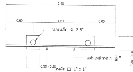
แบบแสดงแปลนป้าย มาตราส่วน 1 : 25
