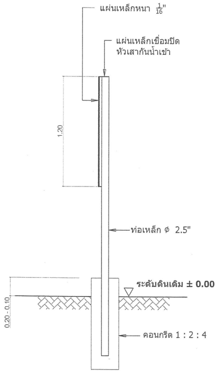
แบบแสดงด้านข้างป้าย มาตราส่วน 1 : 25
