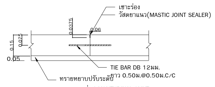
ขยายรอยต่อ LONGITUDINAL JOINT NOT TO SCALE
