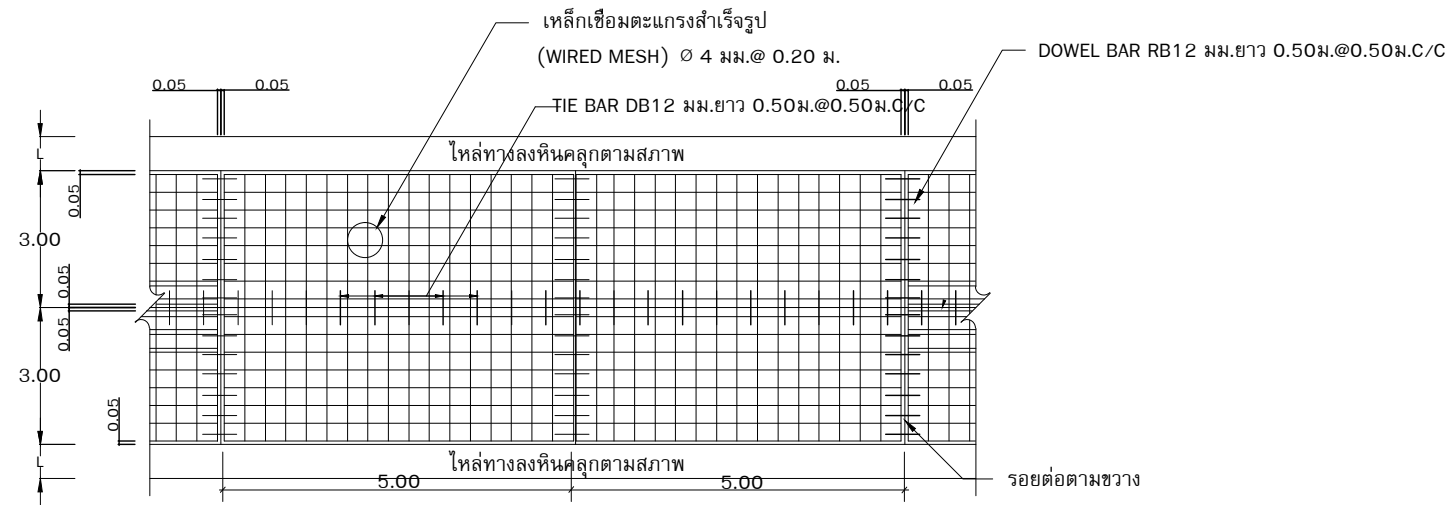
แปลนแสดงการเสริมเหล็กถนน คสล. NOT TO SCALE
